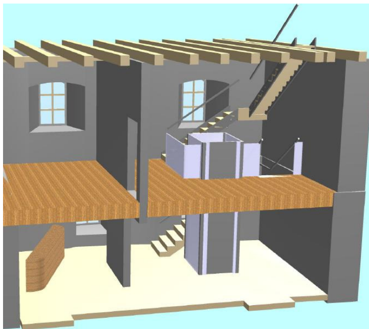
Schema des Ostflügels der Burg mit dem Personenaufzug
